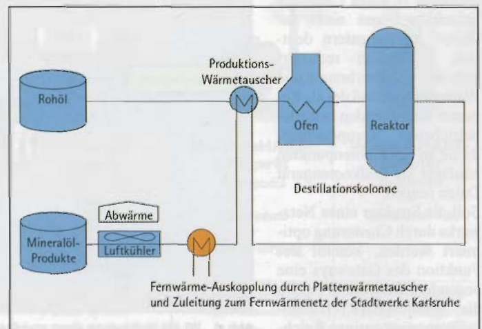
Auskopplung der Prozesswärme als Fernwärme
